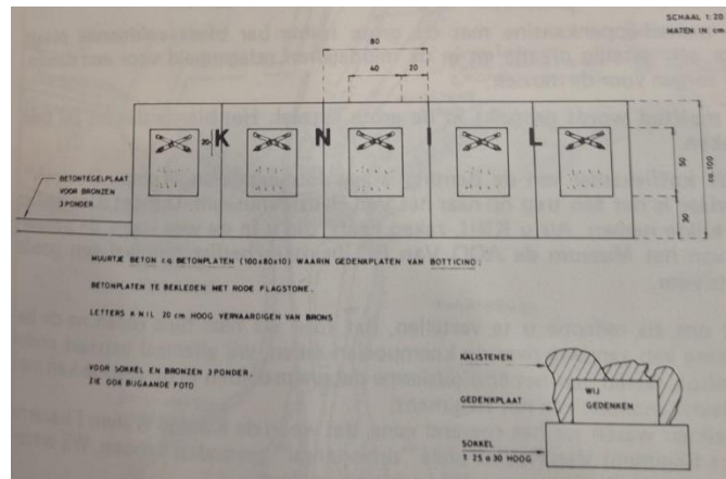
De werktekening van de voorzijde van de muur met de details.
