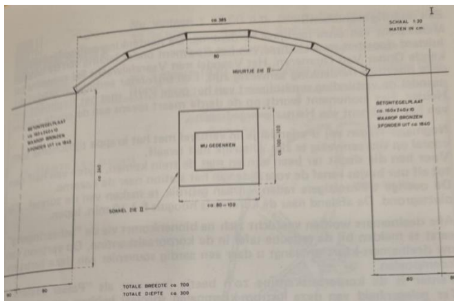
De werktekening met maten zoals die gepresenteerd is aan de leden.
